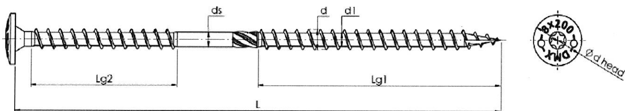
Rysunek 3: Wkręt, typ WKT
