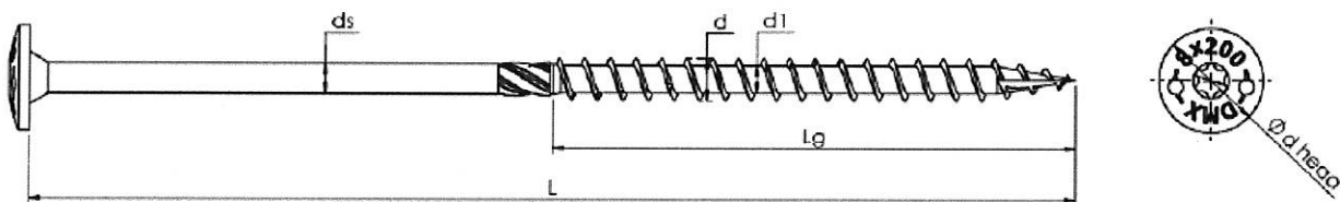
Rysunek 2: Wkręt, typ CT
