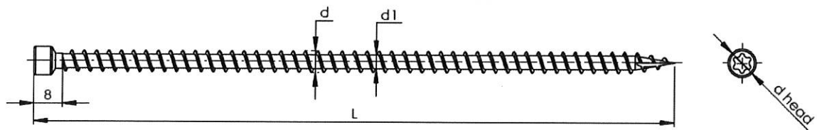
Rysunek 5: Wkręt, typ CPW
