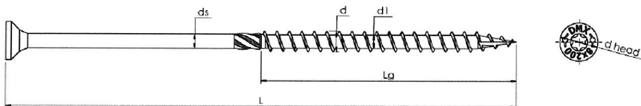
Rysunek 1: Wkręt, typ CS
