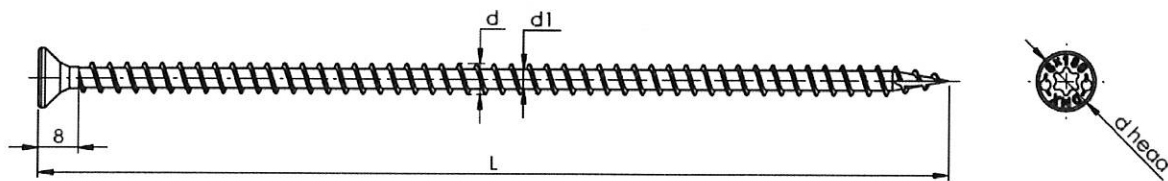
Rysunek 6: Wkręt, typ CPS
