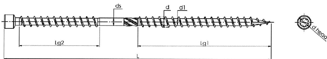
Rysunek 4: Wkręt, typ WKW
